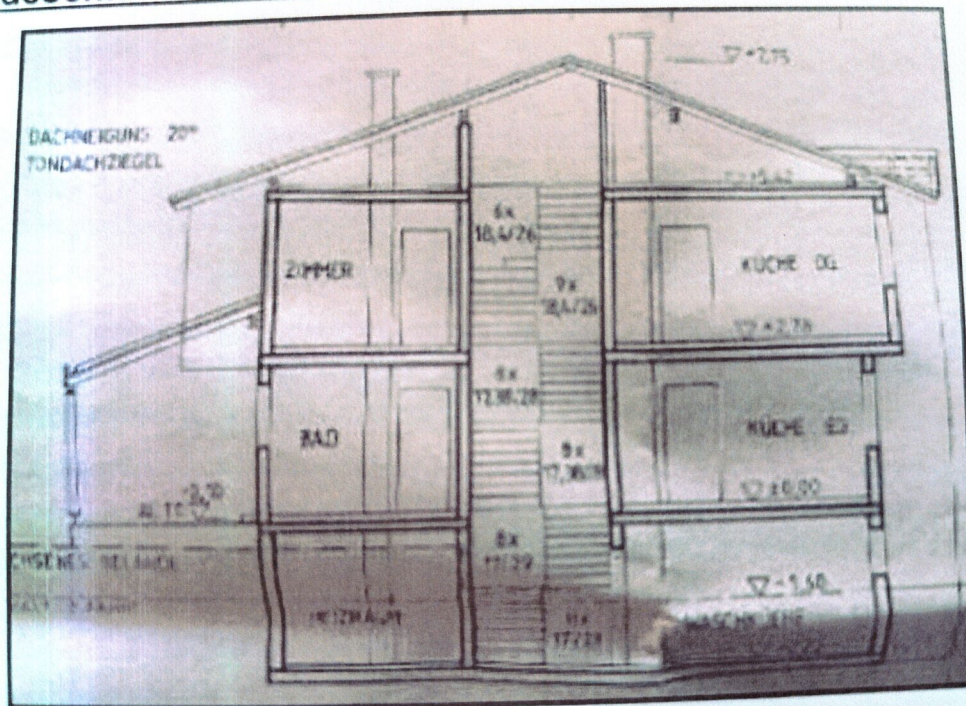
Abbildung 13: Gebäudeschnitt Wohnhaus
